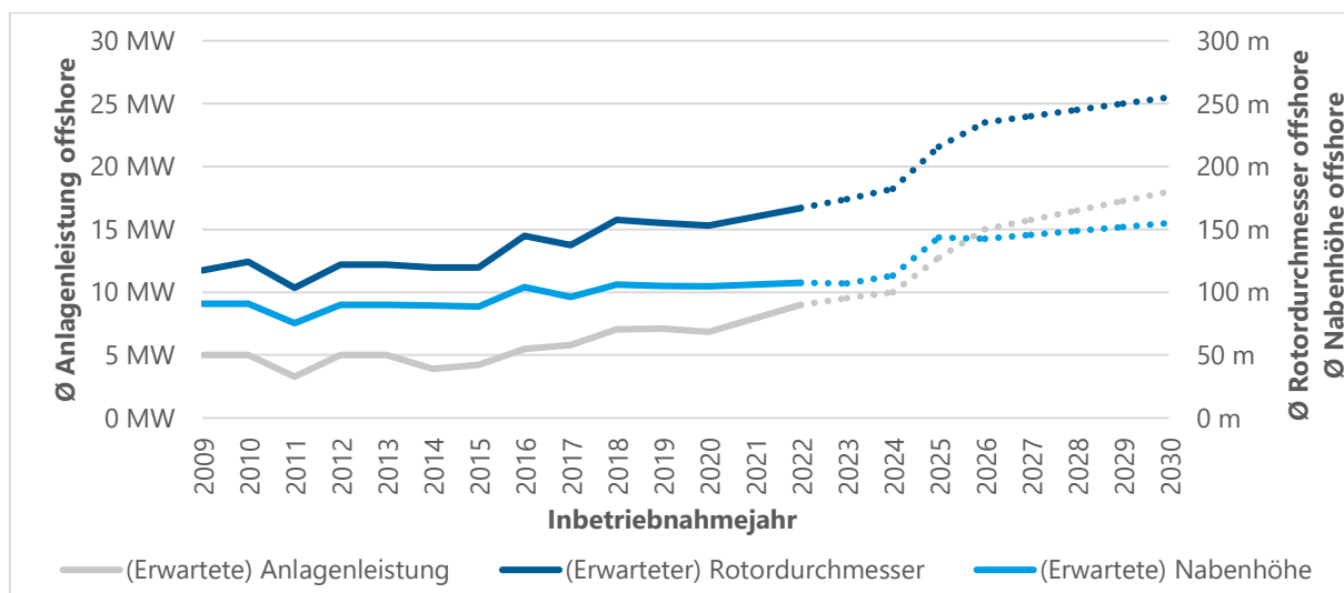
ABBILDUNG 9: (ERWARTETE) ANLAGENENTWICKLUNG OFFSHORE-WINDENERGIE
