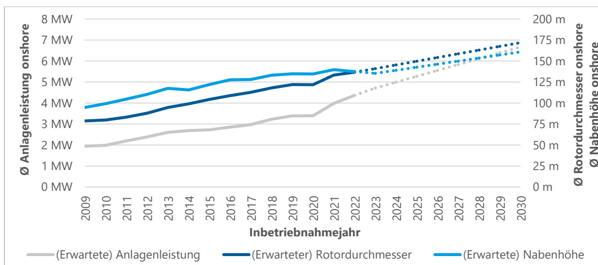
ABBILDUNG 7: (ERWARTETE) ANLAGENENTWICKLUNG ONSHORE-WINDENERGIE
