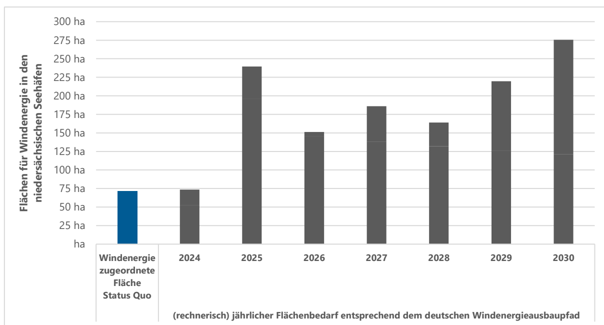
ABBILDUNG 19: JÄHRLICHER FLÄCHENBEDARF DER WINDENERGIEBRANCHE IN DEN NIEDERSÄCHSISCHEN SEEHÄFEN ENTSPRECHEND DEM DEUTSCHEN AUSBAUPFAD
