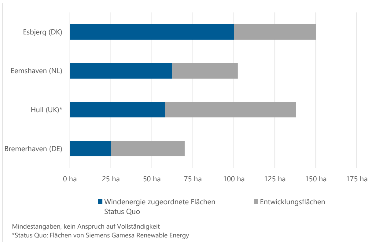
ABBILDUNG 18: FLÄCHENSITUATION IN AUSGEWÄHLTEN WEITEREN NORDSEEHÄFEN IM HINBLICK AUF DIE WINDENERGIE
