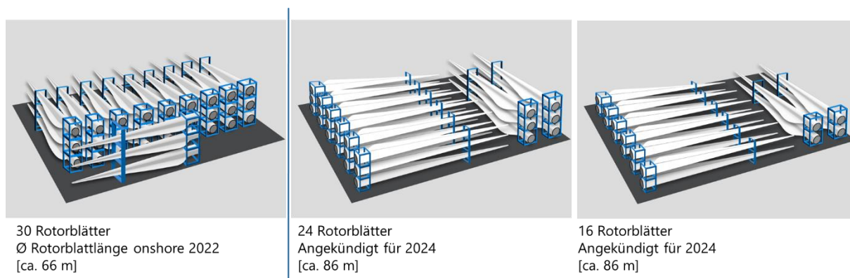
ABBILDUNG 21: EXEMPLARISCHE VISUALISIERUNG DER AUSWIRKUNG VON KOMPONENTEN-ENTWICKLUNGEN AUF DEN FLÄCHENBEDARF
